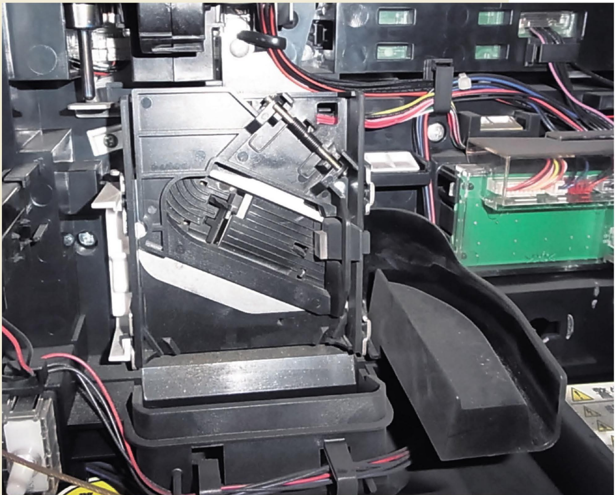
未だに続いているメダルセレクターのカバー欠損事案
