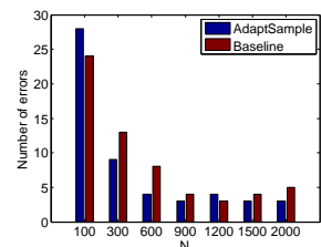
(d) Number of errors w.r.t. number of permutations N
