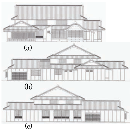
図2 本陣立面図 (a) 北面、(b) 西面、(c) 東面
