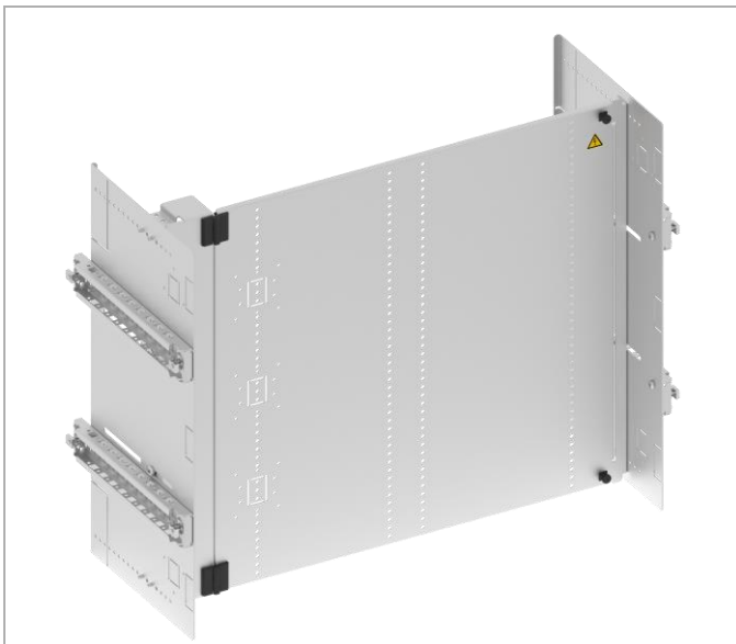
Steuerfach schwenkbar
