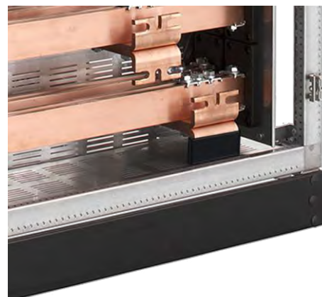
Isolierkappe 773-221-xxx auf Anschlusswinkel
