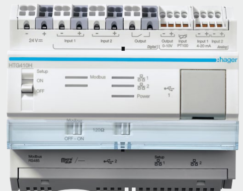
Serveur de surveillance de l'énergie (Modbus Master)
