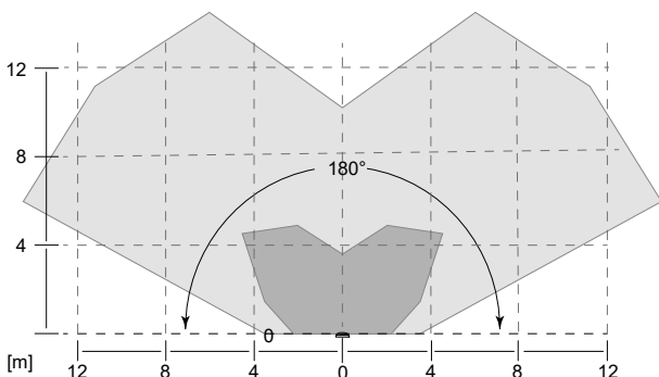
Zone de détection du détecteur de mouvement pour une hauteur de montage nominale d'1,1 m
