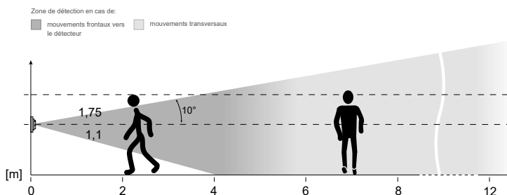
Zone de détection du détecteur de mouvement pour une hauteur de montage nominale d'1,1 m
