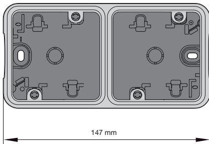
Afbeelding 17: Opbouwbehuizing 2-voudig
