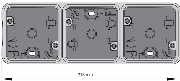
Afbeelding 18: Opbouwbehuizing 3-voudig
