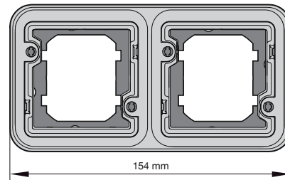
Afbeelding 21: Afdekraam 2-voudig voor inbouwmontage
