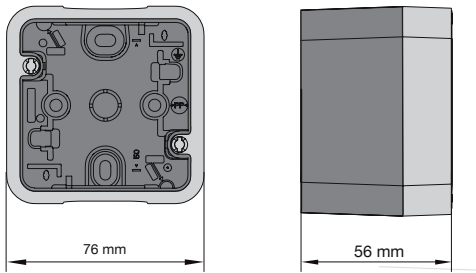
Afbeelding 16: Opbouwbehuizing 1-voudig
