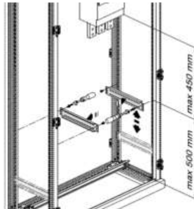
Montagepositie diepteprofielrails
