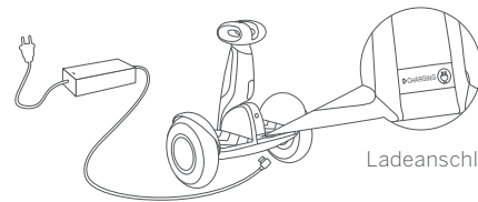
Öffnen Sie die Gummikappe
