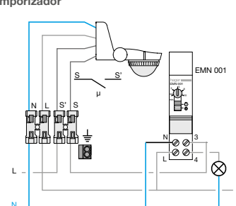
Temporizador
