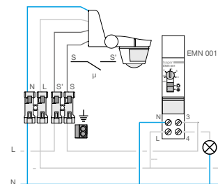
Temporizador
