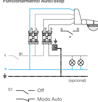
Funcionamiento Auto/Stop
