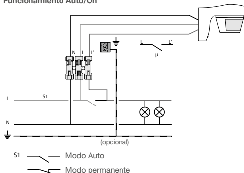
Funcionamiento Auto/On
