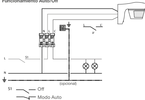
Funcionamiento Auto/Off
