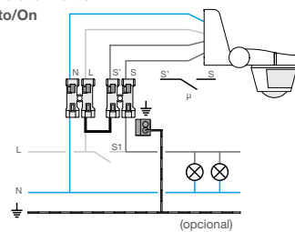
Funcionamiento Auto/On
