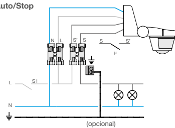
Funcionamiento Auto/Stop
