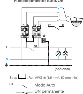
Temporizador
