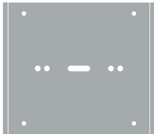
VESA-Halterung
