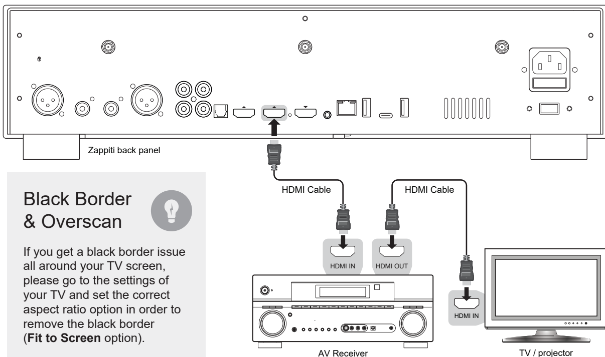
AV Receiver
