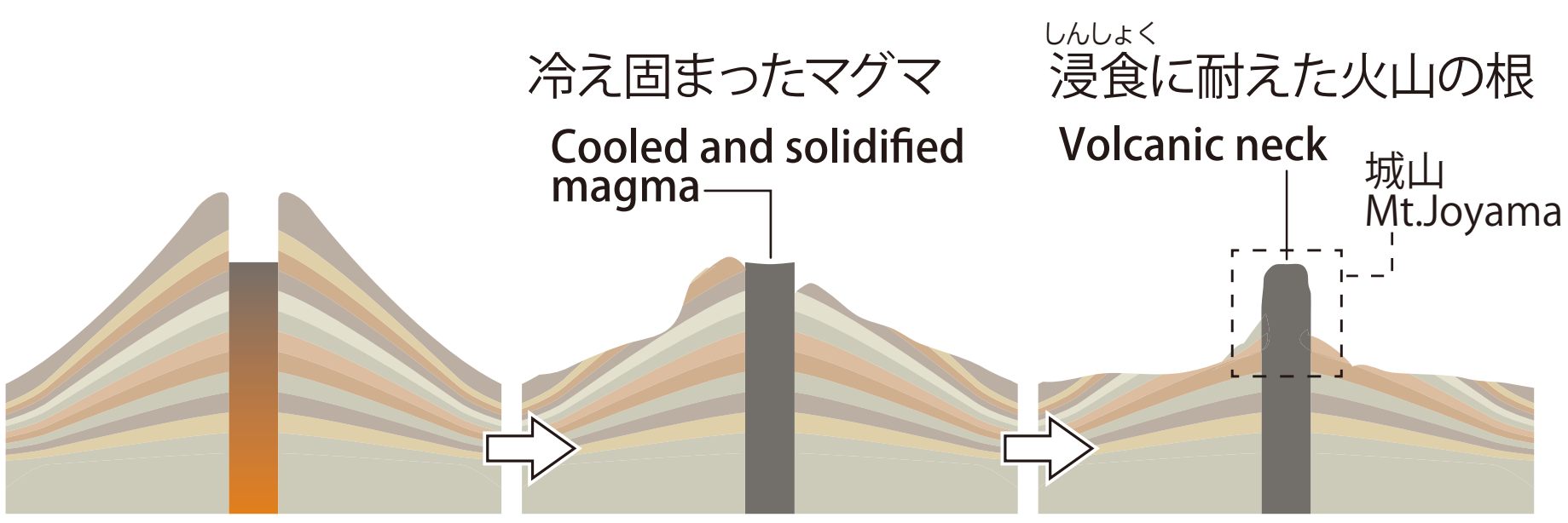
「火山の根」のでき方 Formation of volcanic neck
