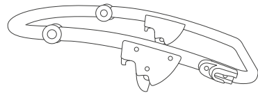
1 x XL basket frame XL Einkaufskorbrahmen
